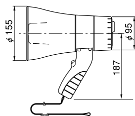
外観寸法図 (単位mm)
